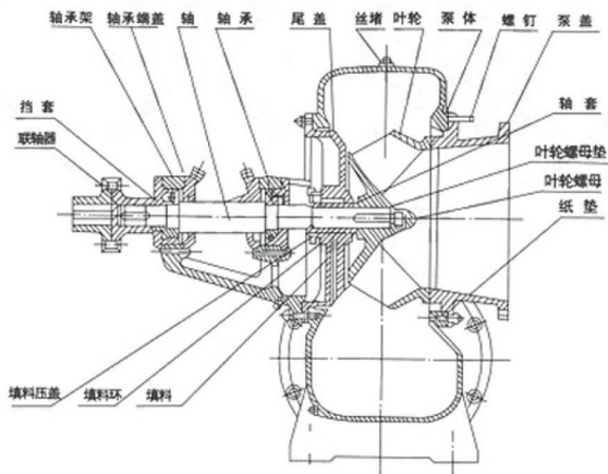
图2 400~800HW型泵结构图(650HW-5、-7、-10型泵的出水方向与图示相反一向泵进口看、叶轮为顺时针旋转)
