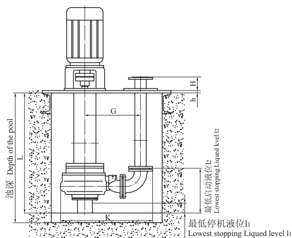
YW系列泵外形安装尺寸表 YW series pump installation dimension
